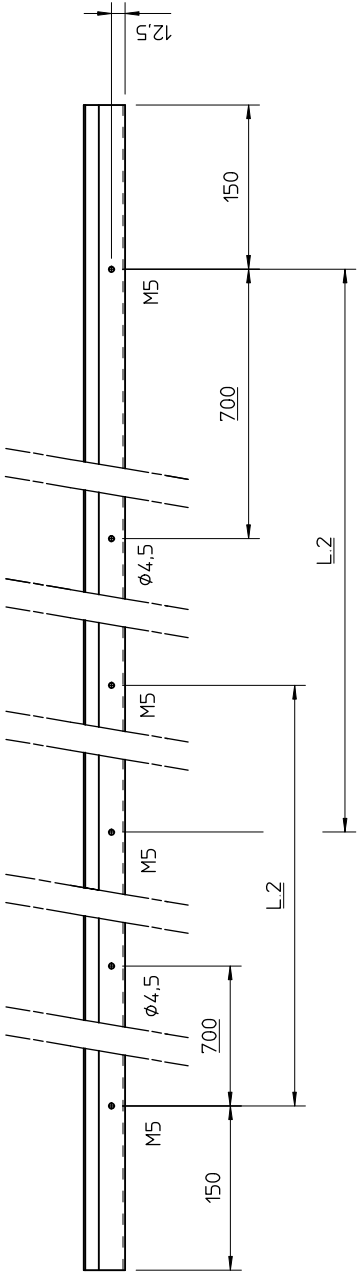
aanzicht A
