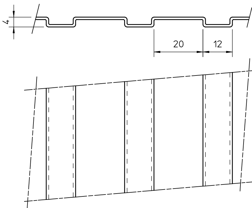
detail profiel schaal 1:1
