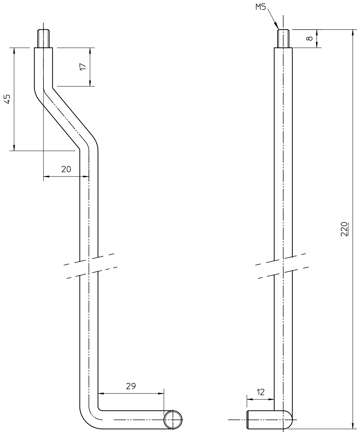
afschuining 0.5 x 45°
